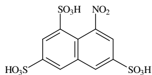
Nitro-T-acid
