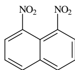
1,8-Dinitronaphtalene
