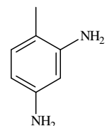
2,4-Diaminotoluene
