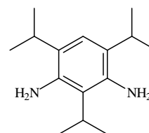
2,4,6-Triisopropylbenzene-1,3-diamine
