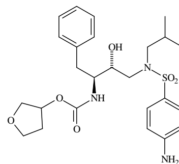
(3S)-Tetrahydro-3-furyl-N-[(1S,2R)-3-(4-amino-N-isobutyl-benzenesulfonamido)-1-benzyl-2-hydroxypropyl]carbamate
