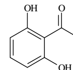
Acetylresorcinol
